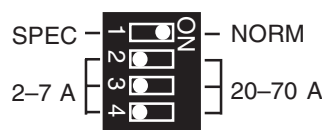
DIL-omkopplare
