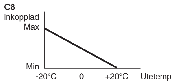
Fig 10. Exempel på styrning från Utetemp-kompensator
