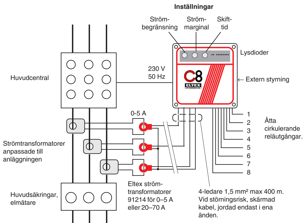
FIG 1. Systemöversikt
