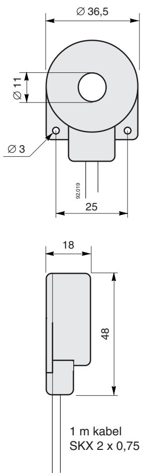
Fig 3 Eltex strömtrafo 91214
